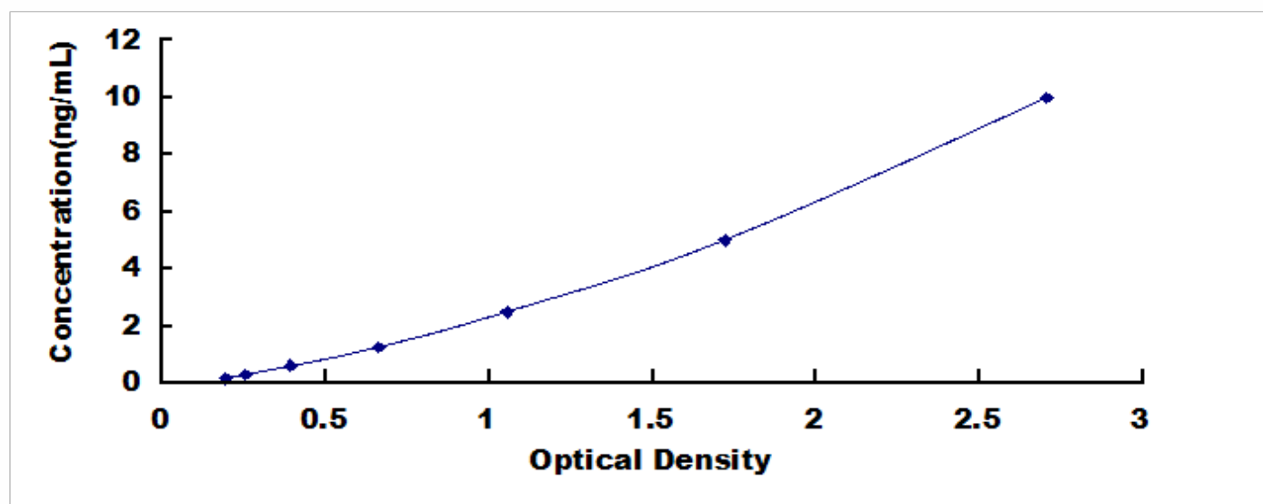
人 Corin 蛋白 (CRN) 检测试剂盒标准曲线
