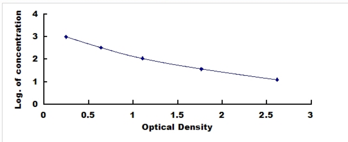
猪促肾上皮质激素释放激素 (CRH) 检测试剂盒标准曲线
