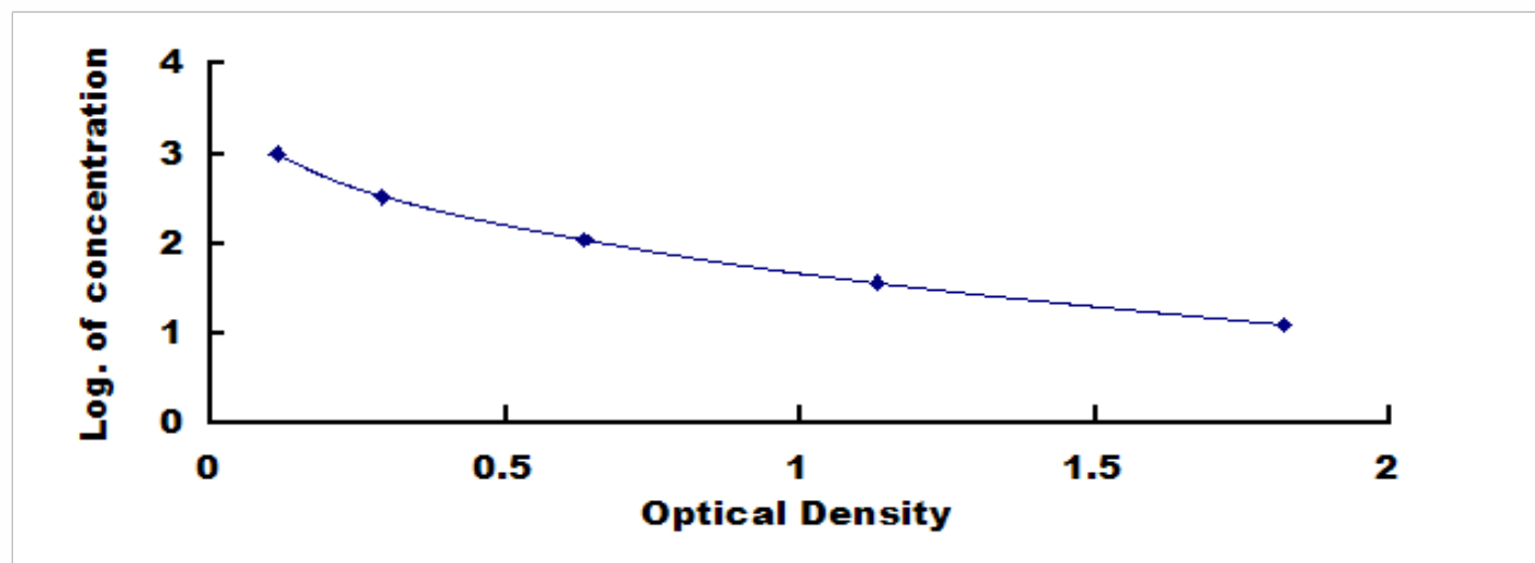
人促肾上腺皮质激素释放激素 (CRH) 检测试剂盒标准曲线
