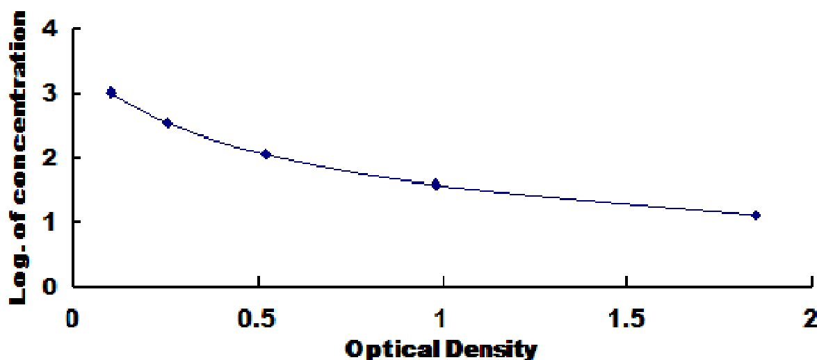
小鼠促肾上腺皮质激素释放激素(CRH)检测试剂盒标准曲线
