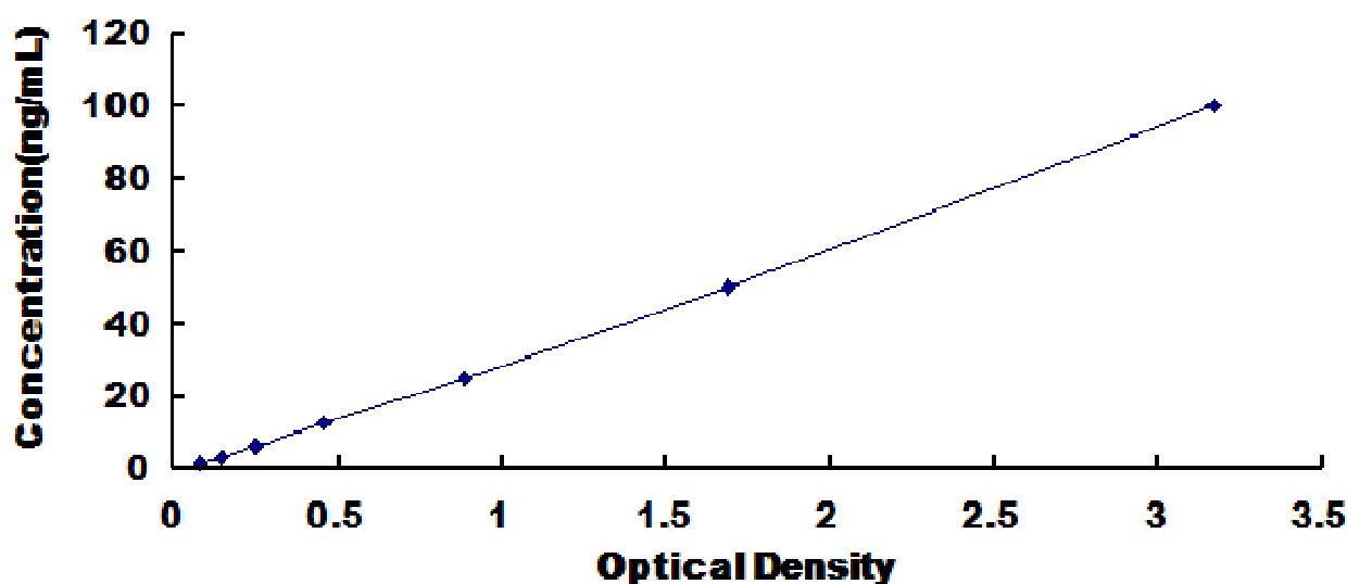
小鼠肌酸激酶(CKM)检测试剂盒标准曲线
