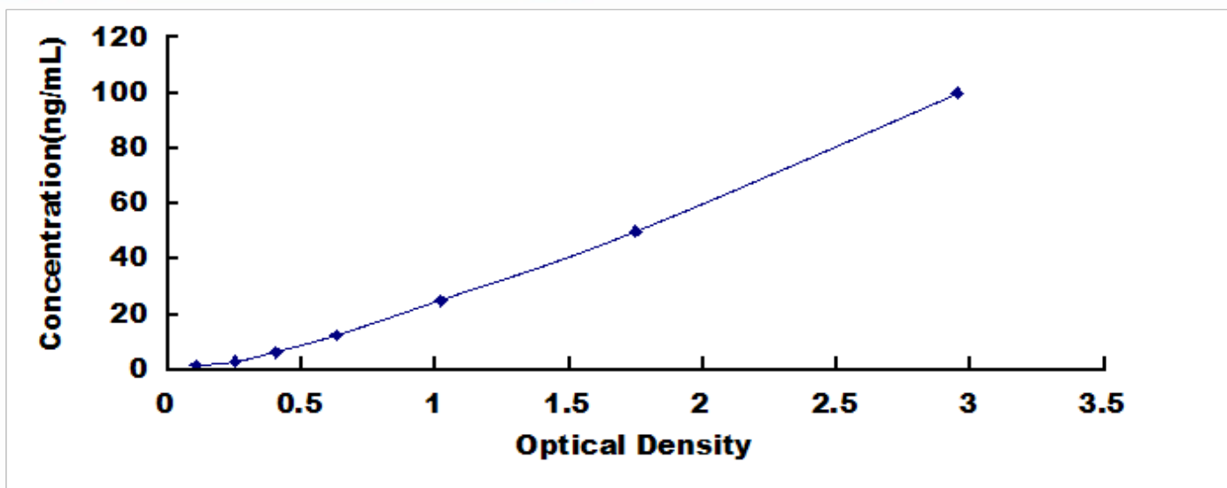
小鼠肌酸激酶(CKM)检测试剂盒标准曲线
