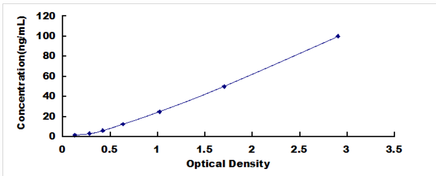
大鼠肌肌酸激酶 (CKM) 检测试剂盒标准曲线
