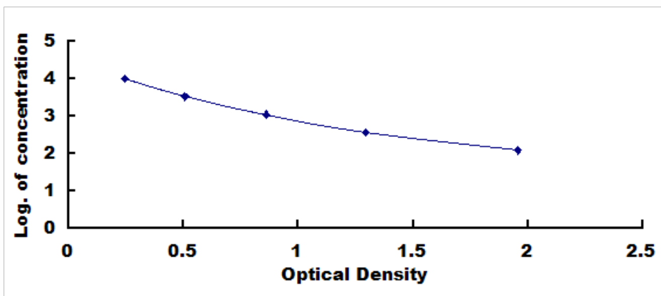
大鼠 I 型胶原交联羧基端肽 (CTX I) 检测试剂盒标准曲线
