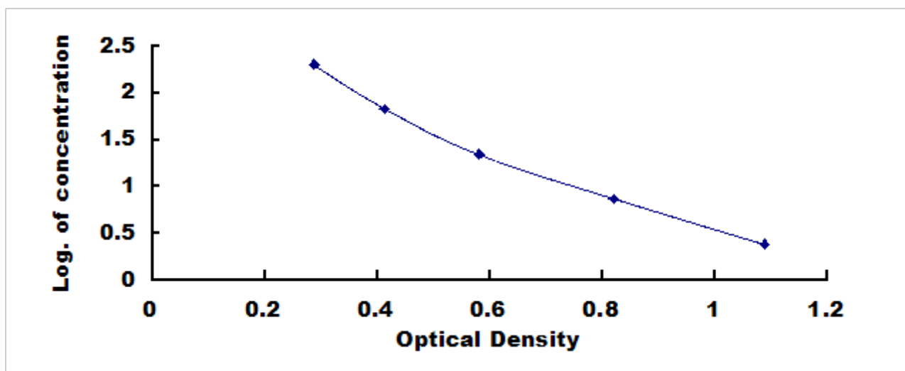
人 I 型胶原交联氨基端肽 (NTX I) 检测试剂盒标准曲线
