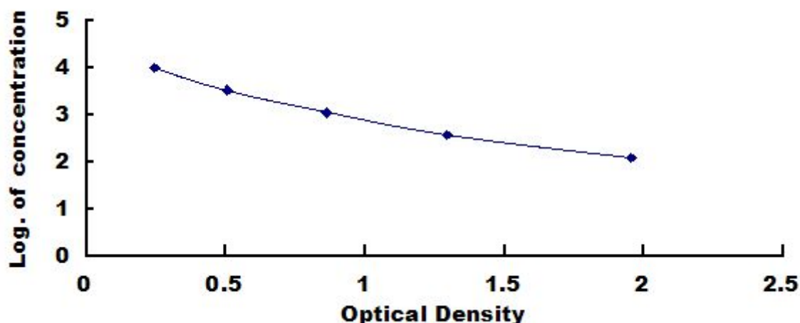
氰钴胺素 (CNCb1) 检测试剂盒标准曲线
