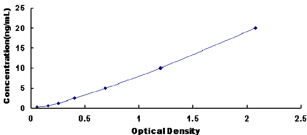
人细胞周期素 D1 (CCND1) 试剂盒标准曲线
