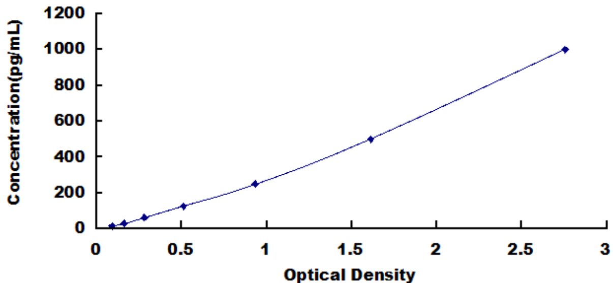
人细胞周期素 D2 (CCND2) 检测试剂盒标准曲线
