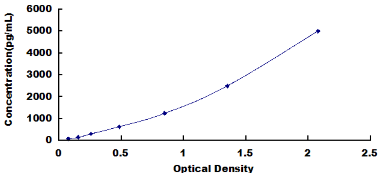
人细胞周期素 Y (CCNY) 检测试剂盒标准曲线
