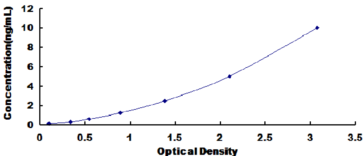
大鼠细胞胱硫醚 \gamma 裂解酶(CSE)检测试剂盒标准曲线
