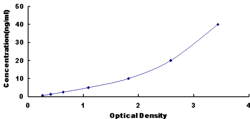
图 1: 大鼠半胱氨酸蛋白酶抑制剂(Cys-C)试剂盒标准曲线
