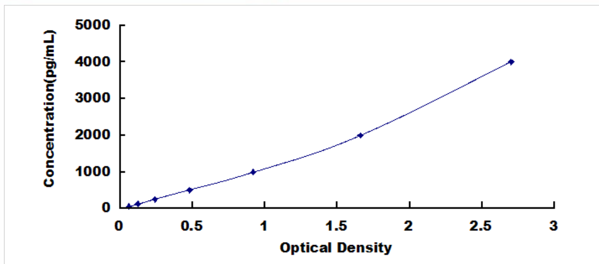
人半胱氨酸丰富血管生成诱导因子 61 (CYR61) 检测试剂盒标准曲线
