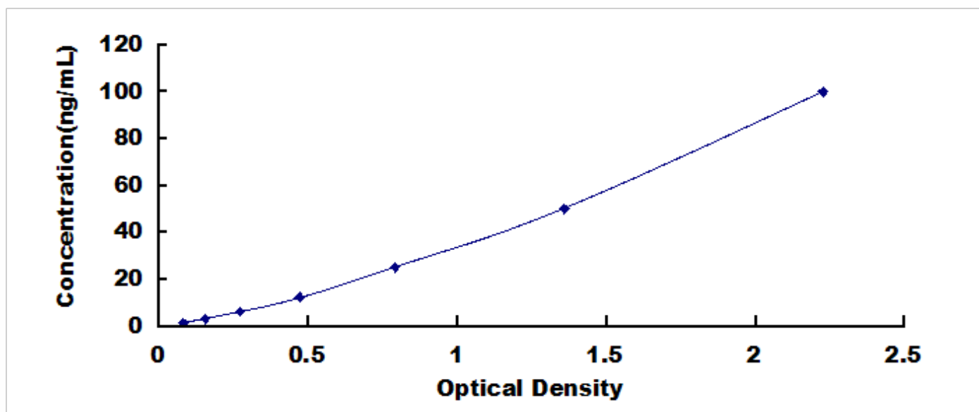
大鼠细胞色素 C (CYCS) 检测试剂盒标准曲线
