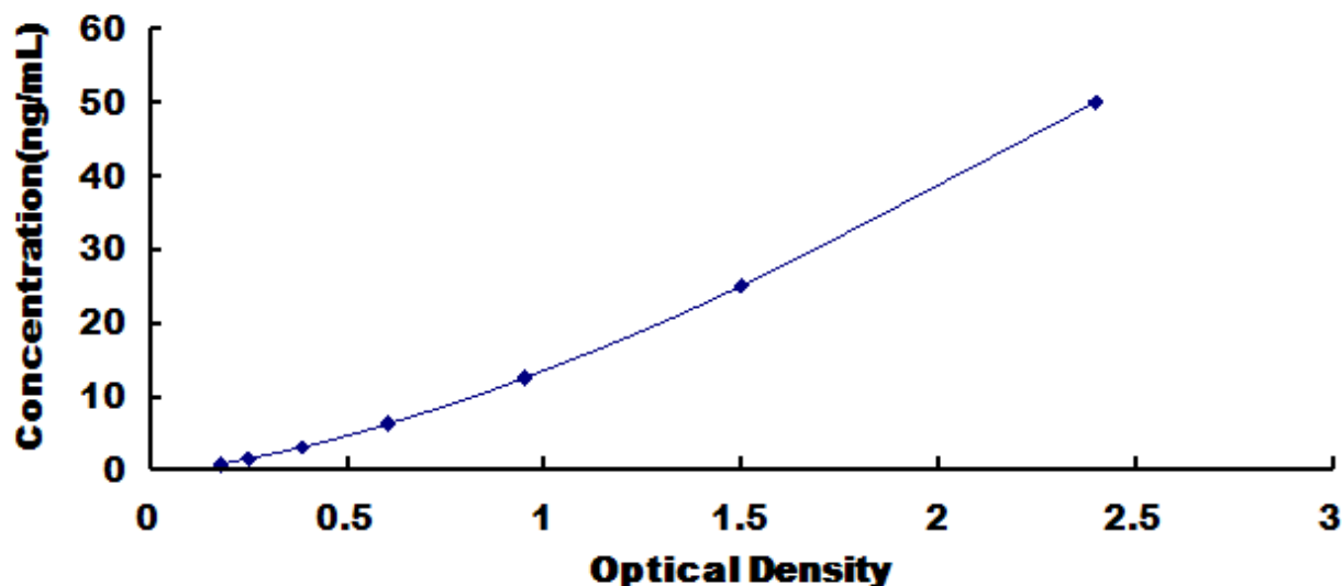
大鼠细胞色素 P450 家族成员 11B1 (CYP11B1) 检测试剂盒标准曲线
