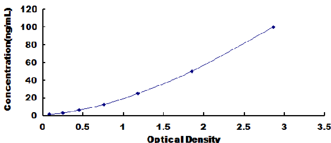
大鼠细胞色素 P450 家族成员 2D6(CYP2D6)试剂盒标准曲线
