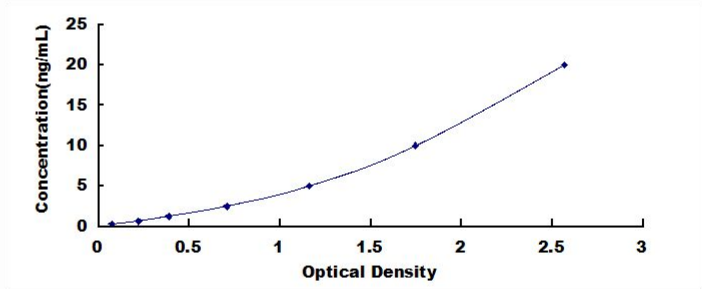
人细胞色素 P450 家族成员 3A4 (CYP3A4) 检测试剂盒标准曲线
