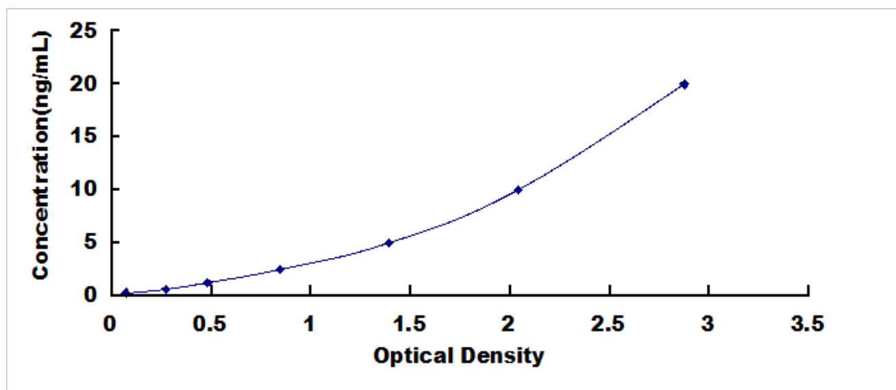
小鼠细胞色素 P450 家族成员 7A1 (CYP7A1) 检测试剂盒标准曲线
