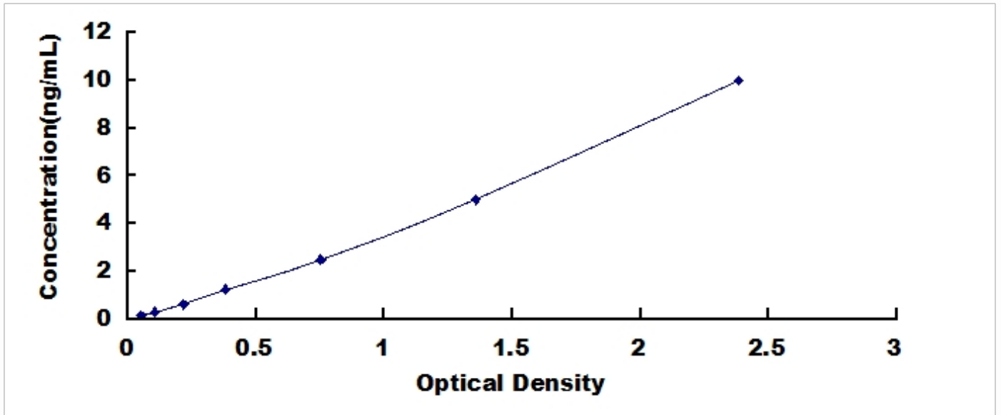
人细胞色素 b-245 \beta 肽 (CYB \beta ) 检测试剂盒标准曲线
