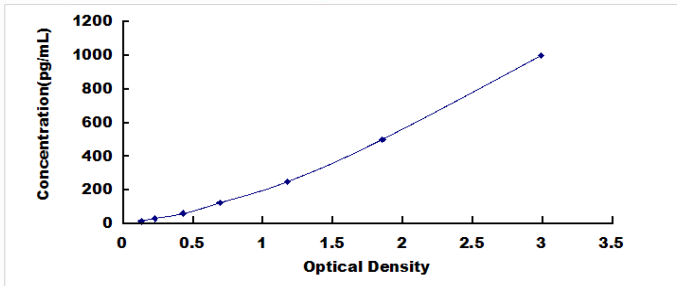
人细胞因子受体样因子 1 (CRLF1) 检测试剂盒标准曲线
