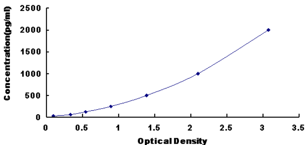
图 1: 人衰变加速因子(DAF)试剂盒标准曲线
