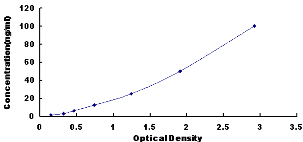
图 1: 猪 \beta 防御素 1(DEF \beta 1)试剂盒标准曲线
