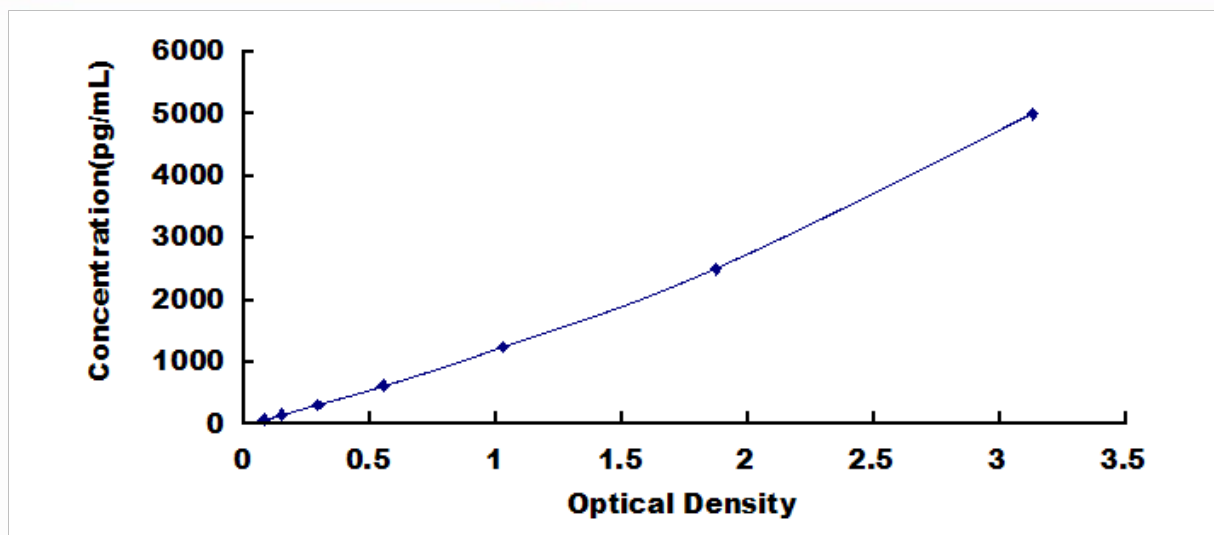
人脱氧核糖核酸酶 I (DNASE1) 检测试剂盒标准曲线
