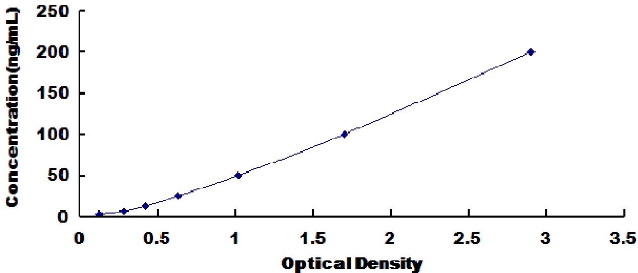
大鼠二胺氧化酶(DAO)检测试剂盒标准曲线
