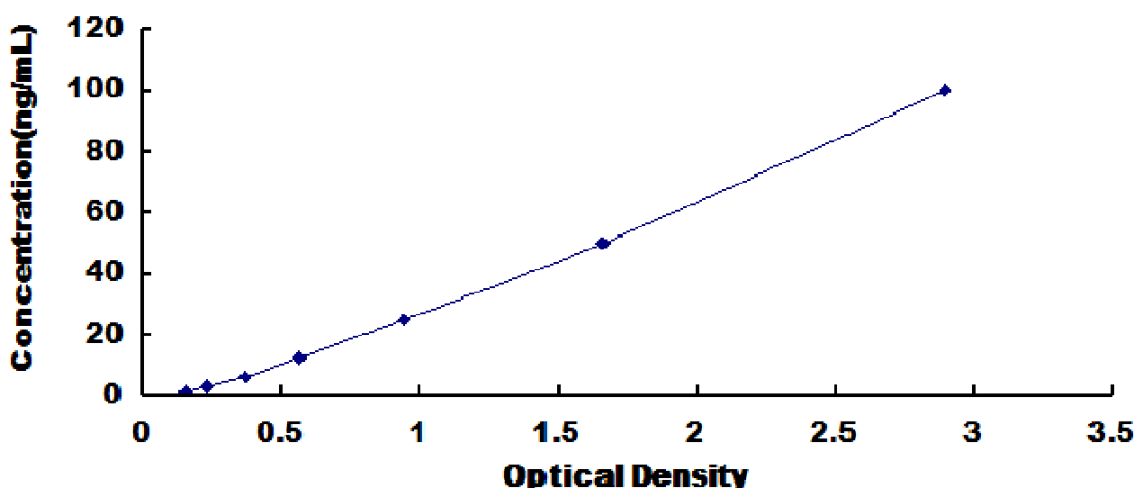
猪二胺氧化酶(DAO)试剂盒标准曲线
