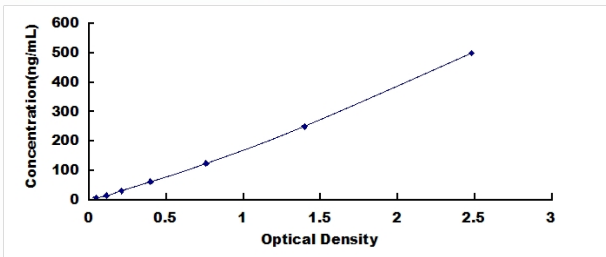
小鼠安定结合抑制因子 (DBI) 检测试剂盒标准曲线
