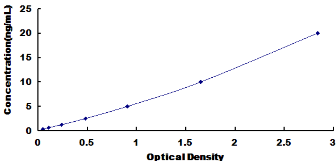
人 Dicer1 酶(DICER1)试剂盒标准曲线
