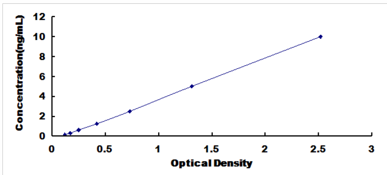
人双肾上腺皮质激素样激酶 1 (DCLK1) 检测试剂盒标准曲线
