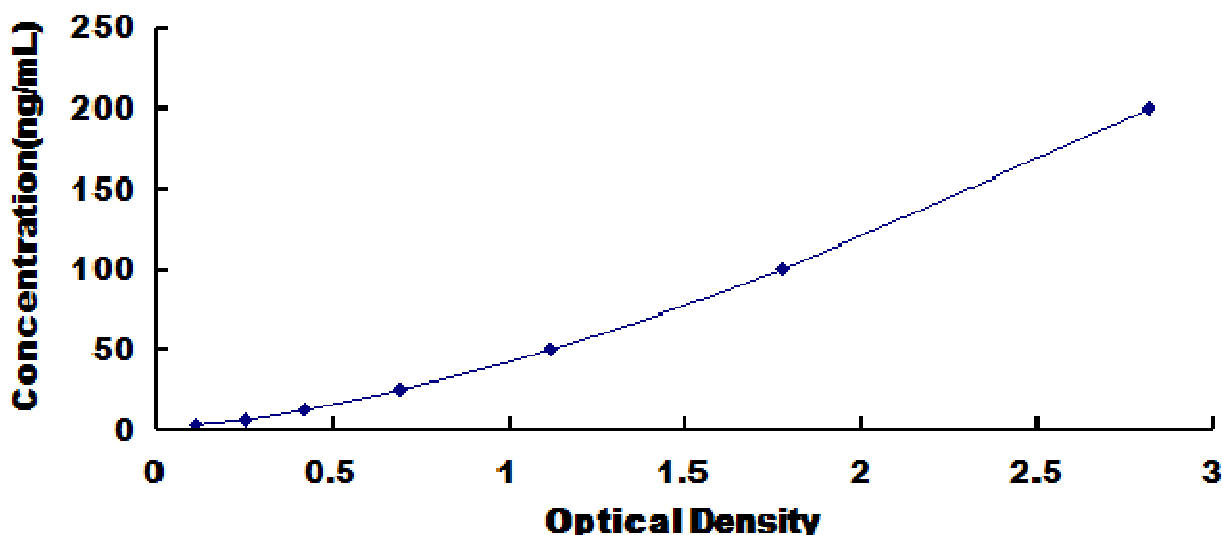
犬中性粒细胞弹性蛋白酶(ELA2)试剂盒标准曲线
