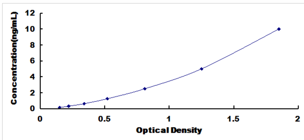
小鼠中性粒细胞弹性蛋白酶(ELA2)检测试剂盒标准曲线
