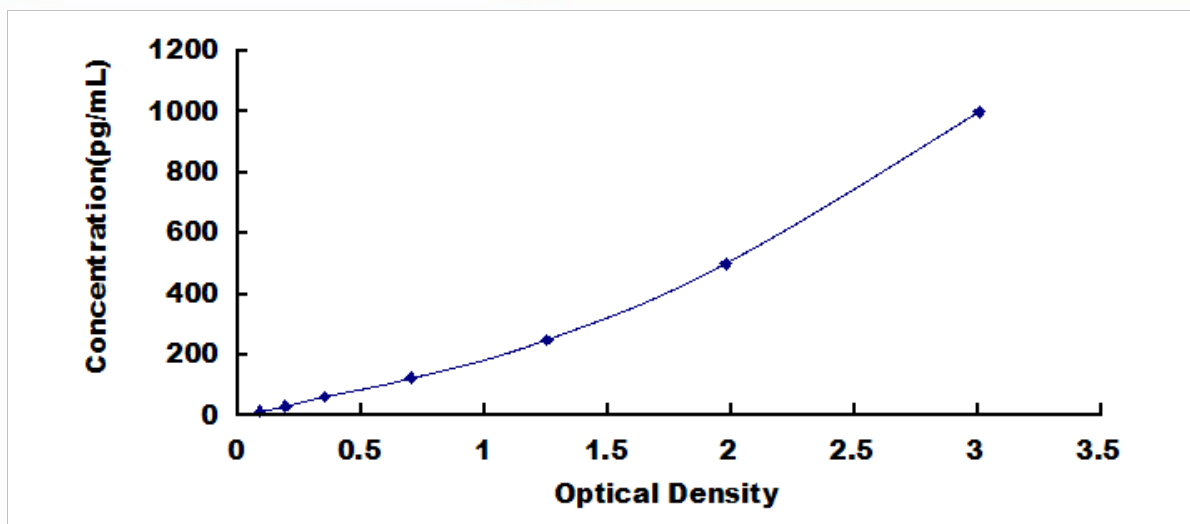
人内皮细胞特异分子 1 (ESM1) 检测试剂盒标准曲线
