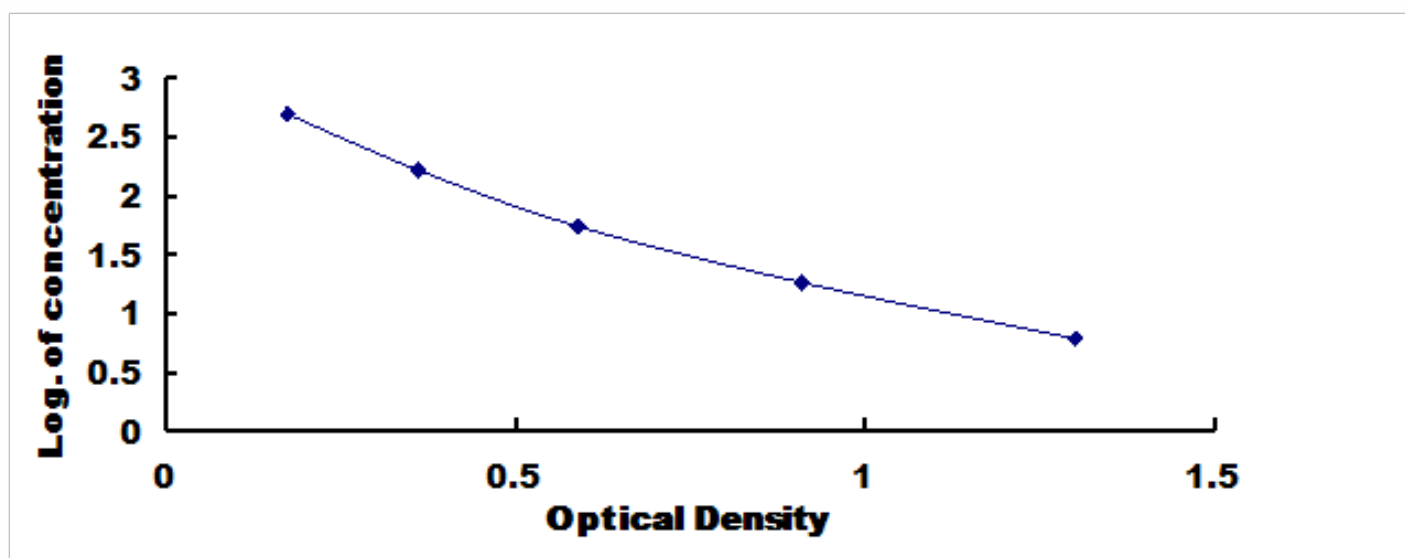
人内皮素 1 (EDN1) 检测试剂盒标准曲线
