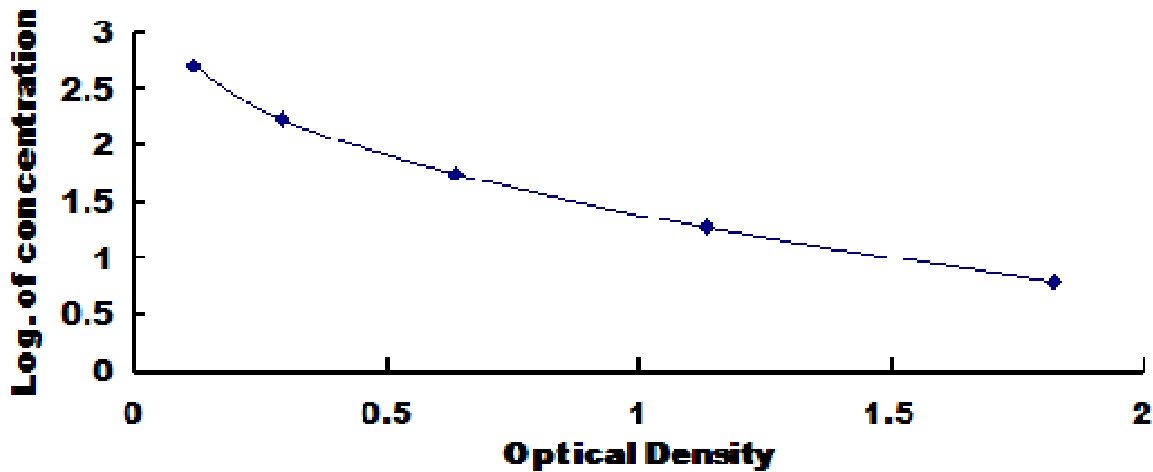
小鼠内皮素 1 (EDN1) 检测试剂盒标准曲线
