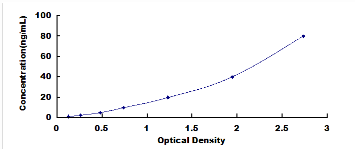
人嗜酸性粒细胞过氧化物酶(EPX)检测试剂盒标准曲线
