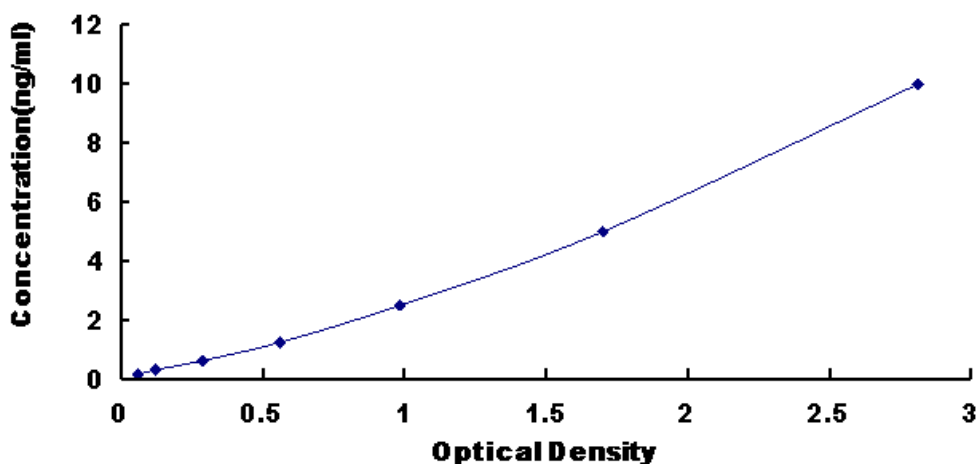
图 1: 人的 Ephrin-A1(EFNA1) 试剂盒标准曲线
