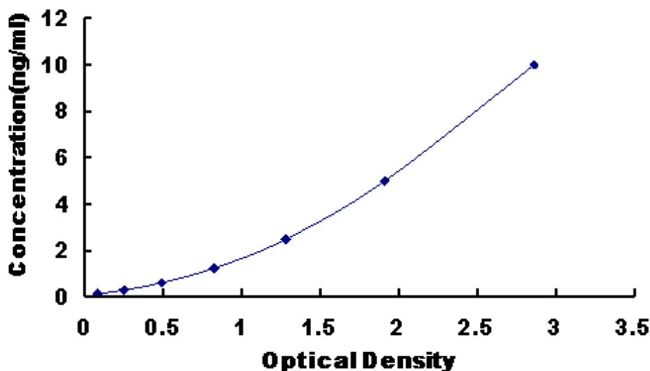
图 1: 人的红细胞生成素受体(EPOR)试剂盒标准曲线
