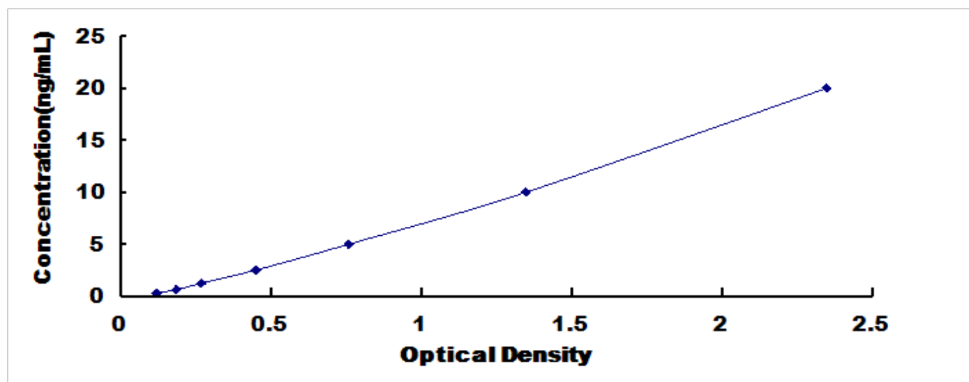
大肠杆菌宿主残留蛋白 (ECP) 检测试剂盒标准曲线
