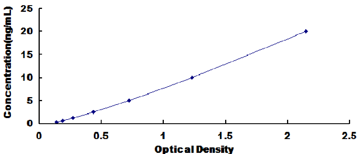
大鼠雌激素受体 \beta (ER \beta )检测试剂盒标准曲线
