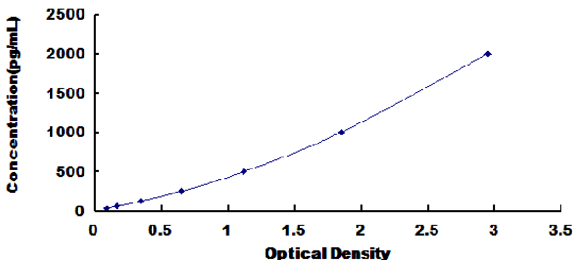
小鼠脂肪细胞型脂肪酸结合蛋白(FABP4)检测试剂盒标准曲线
