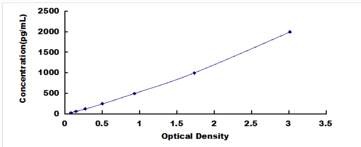
人脂肪细胞型脂肪酸结合蛋白 (FABP4) 检测试剂盒标准曲线
