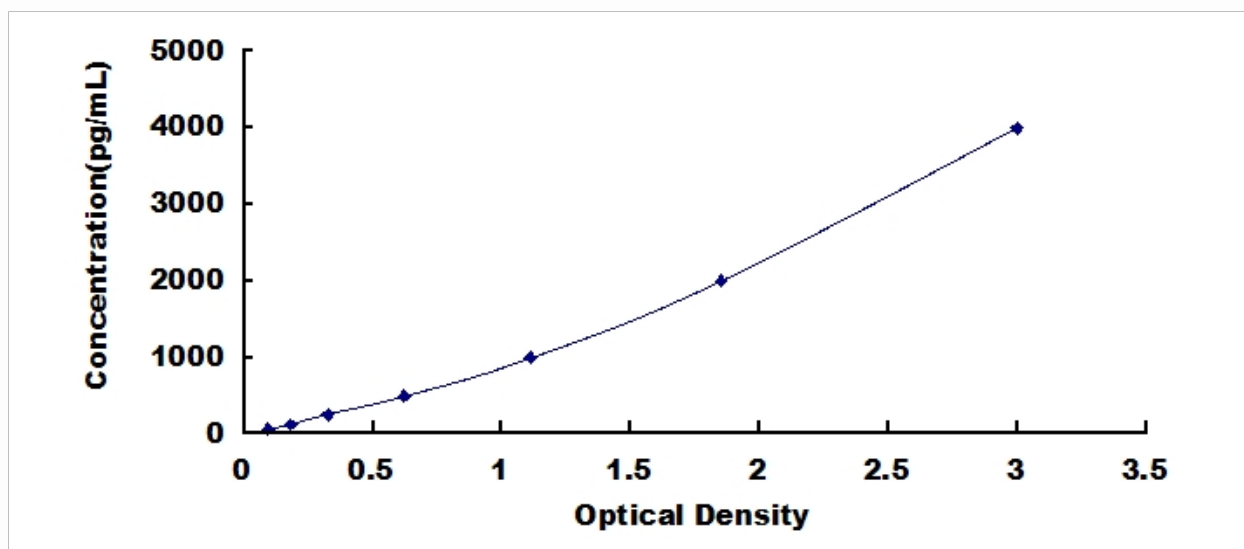
人回肠脂肪酸结合蛋白(FABP6)检测试剂盒标准曲线
