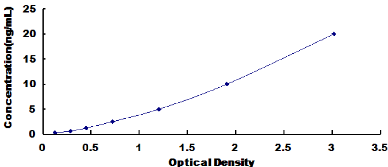
人脂肪酸合酶(FASN)检测试剂盒标准曲线
