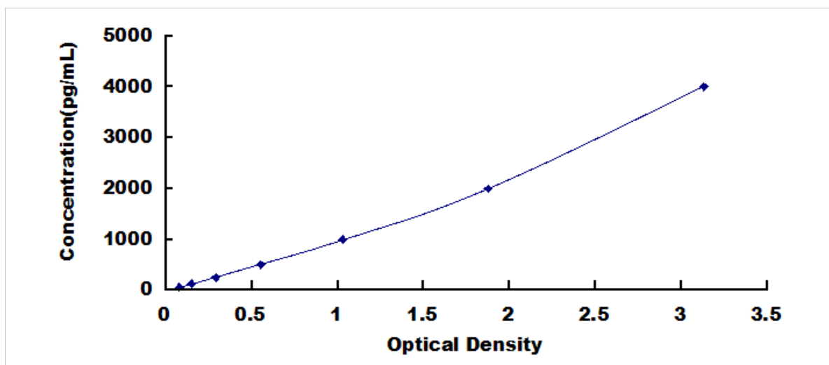
小鼠铁蛋白 (FE) 检测试剂盒标准曲线
