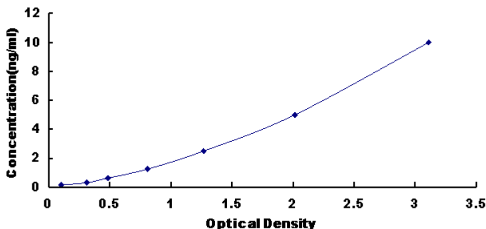
图 1: 大鼠膜铁转运蛋白 Ferroportin(FPN) 试剂盒标准曲线
