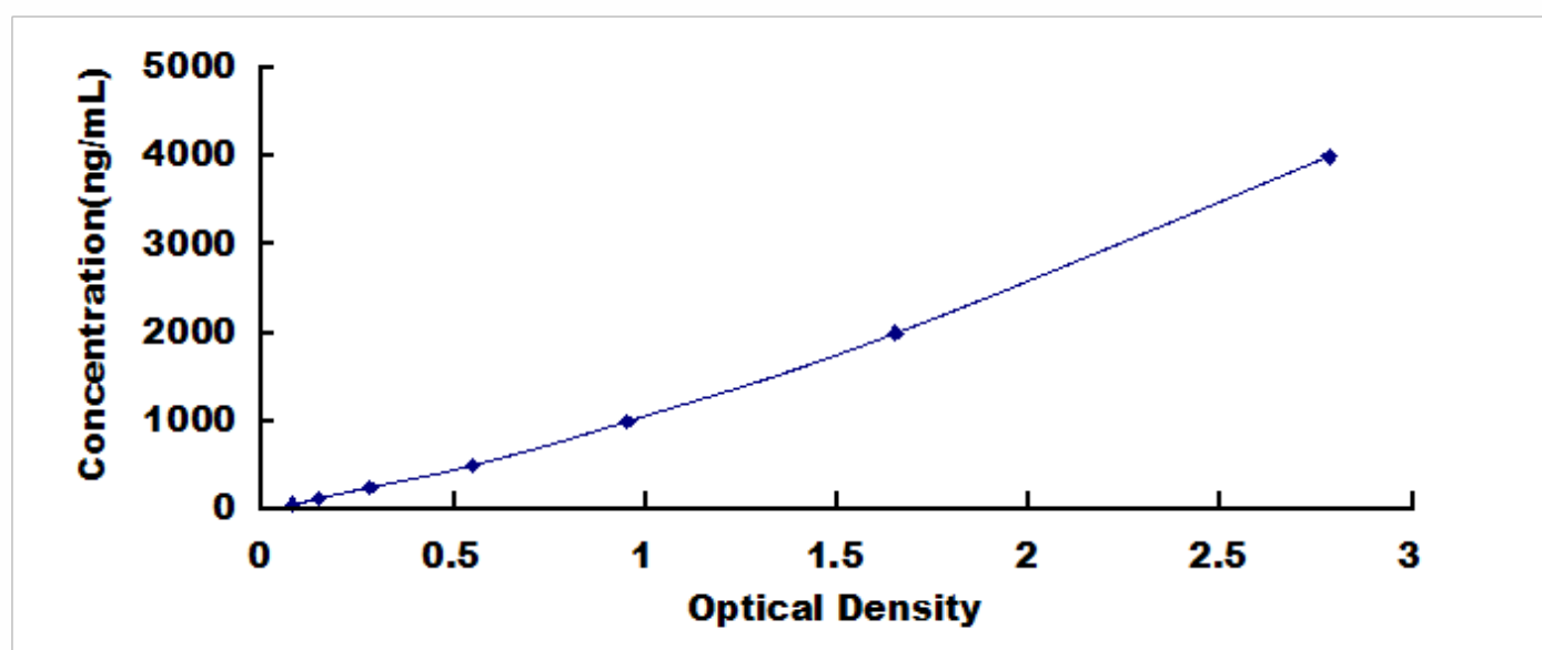
小鼠纤维蛋白原 (FG) 检测试剂盒标准曲线
