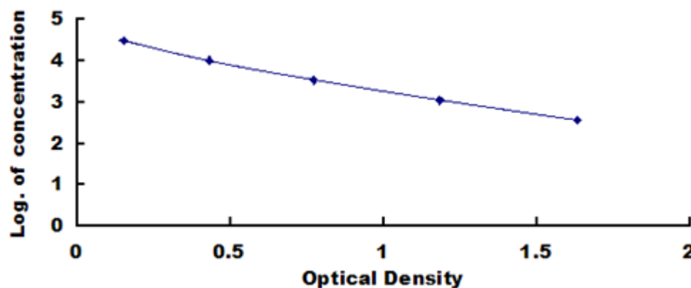
人纤维蛋白肽 B (FPB) 检测试剂盒标准曲线
