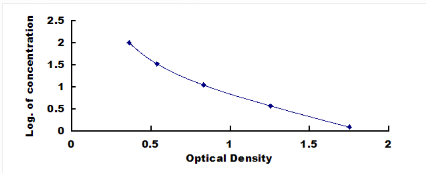
小鼠成纤维细胞生长因子 15 (FGF15) 检测试剂盒标准曲线
